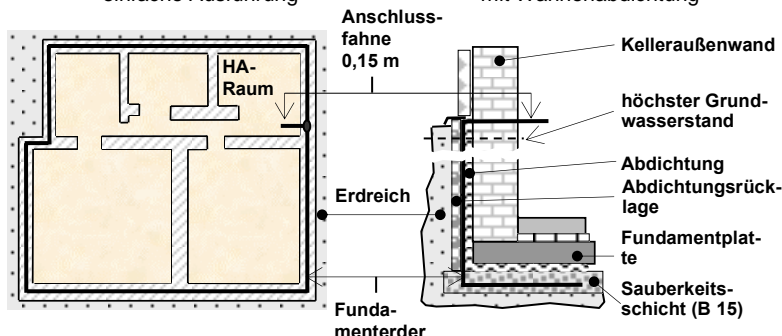
Bild 3 - Beispiele der Anordnung des Fundamenterders im Einzelhaus
